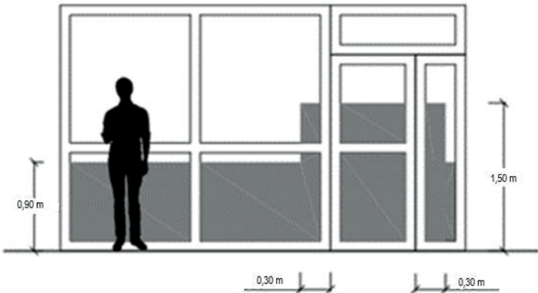
Figura 9. Identificación de áreas con riesgo de impacto en puertas, mamparas y paños fijos
