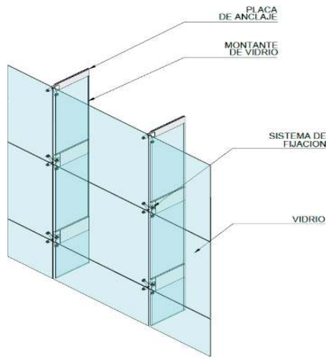
Figura 4. Sistema suspendido
