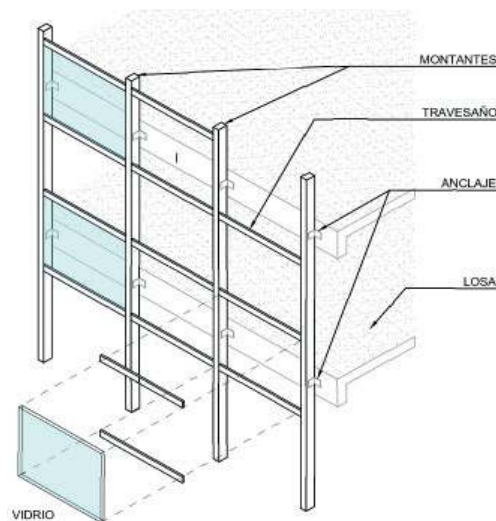
Figura 3. Esquema de fachada con Sistema Stick
