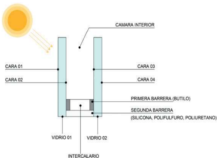
Figura 7. Esquema de un vidrio insulado
