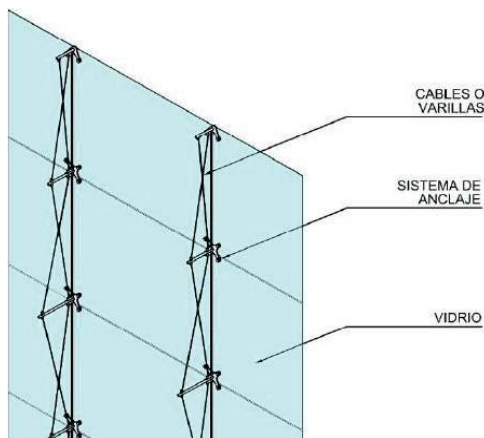
Figura 1. Sistema pretensado
