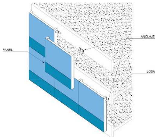
Figura 5. Esquema de fachada con sistema unitizado
