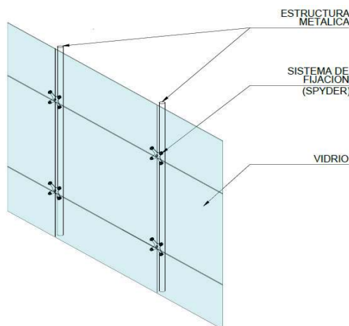
Figura 2. Sistema con arañas (abotonado o spider)
